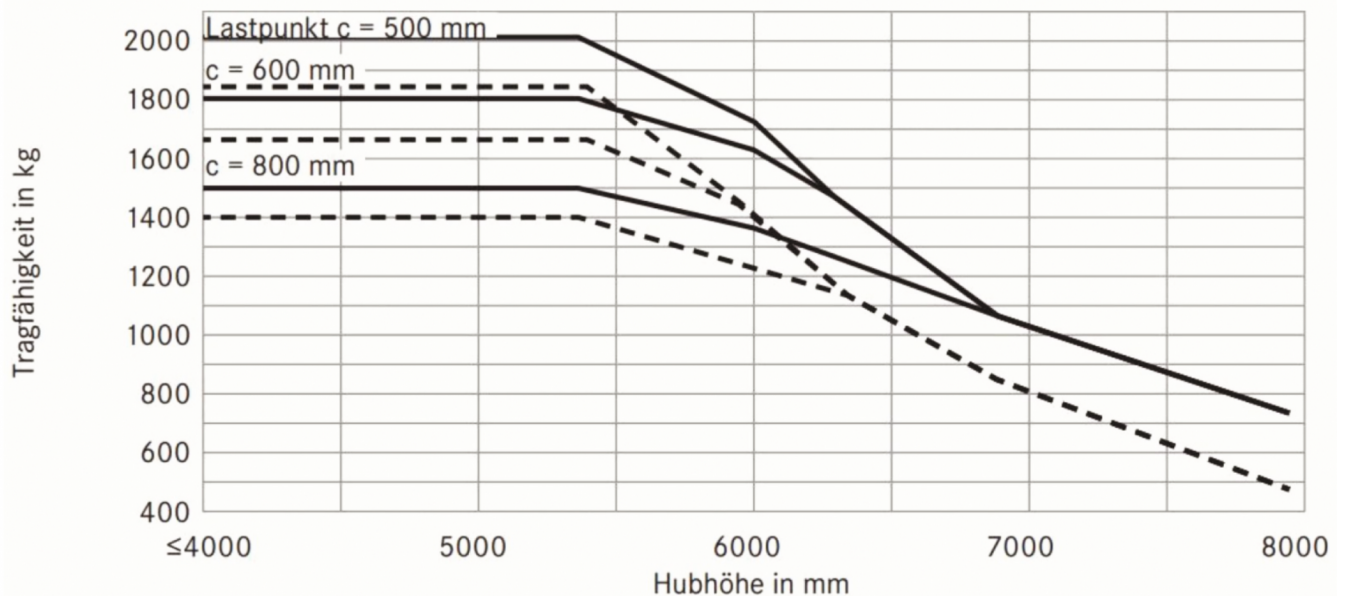
RX 20-20P Dreifach-Hubgerüst Einfach SE-Bereifung
